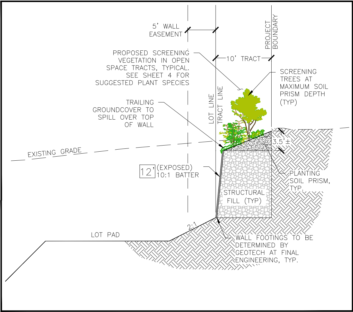
SECTION D-D
